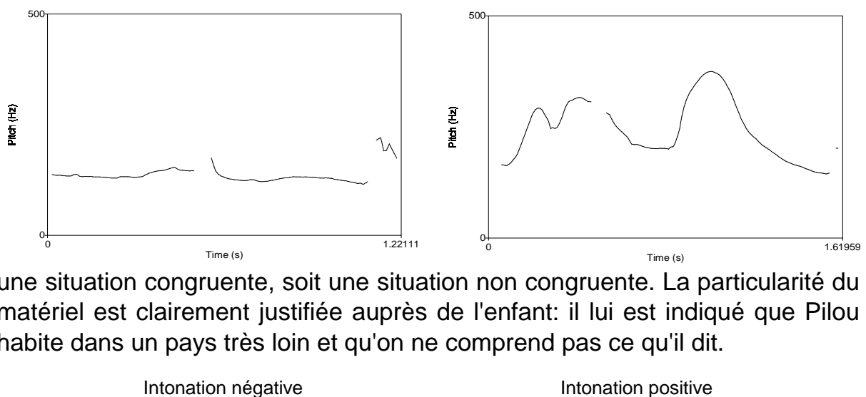
Fig. 2 Contour intonatif (fréquence fondamentale et durée) dans les deux conditions expérimentales.
